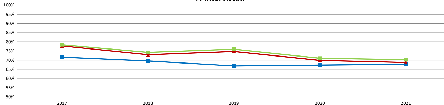
% Intervistati
